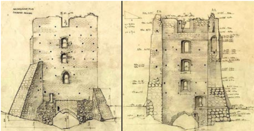
Ryc. 3 i 4. Baszta Szczytówka
